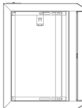
Вид сбоку (без панели)
