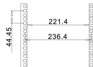
Установочные размеры
