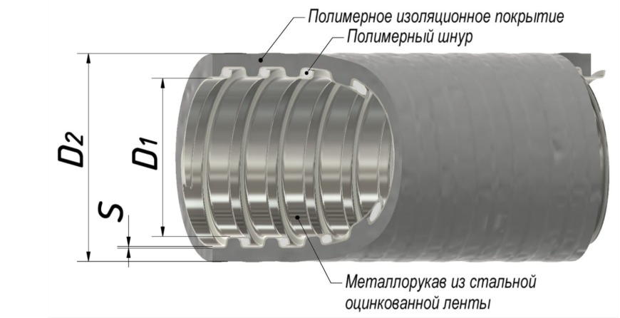
Рисунок 1. Металлорукав типа МПГ нг серый с протяжкой
