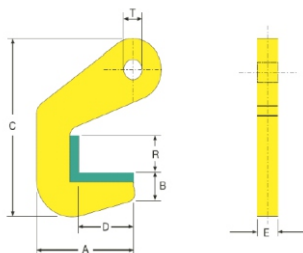
Рисунок 1. Размеры захвата
