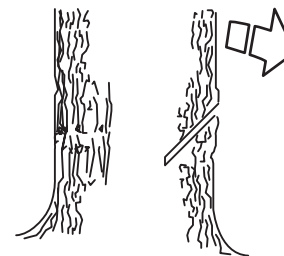
Рисунок 12 — Верхний пропил
