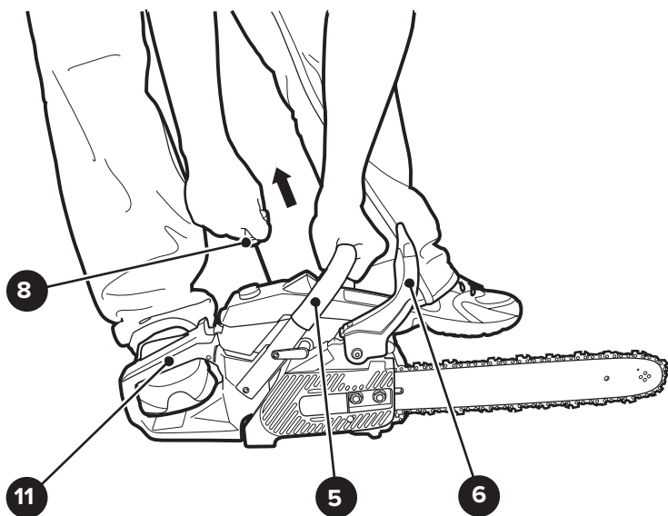
5. Рукоятка передняя 6. Рычаг цепного тормоза
