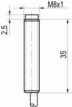
Габаритный чертеж
