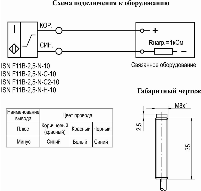
Схема подключения к оборудованию
