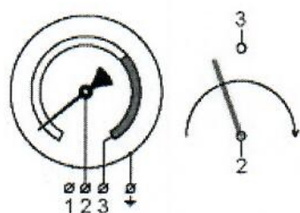
Исполнение I ОЗ (один замыкающий контакт)
