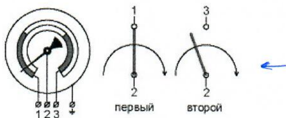
Исполнение V ЛРПЗ (левый размыкающий контакт, правый замыкающий)
