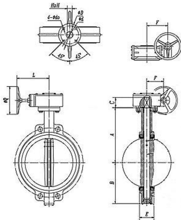
Рисунок 2 - Размеры
