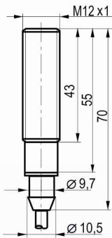
Габаритный чертеж
