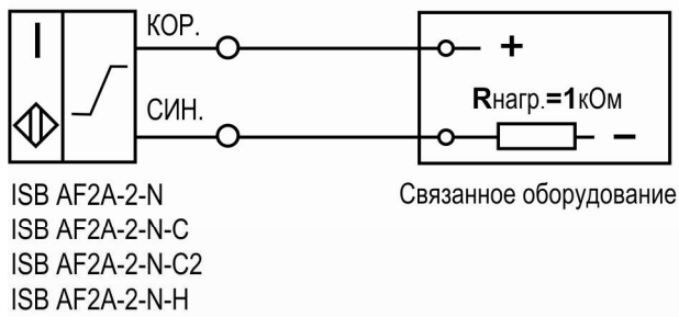
Схема подключения к оборудованию
