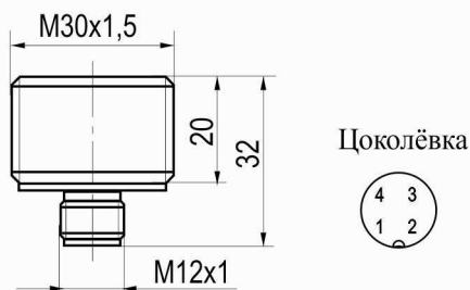
Габаритный чертеж
