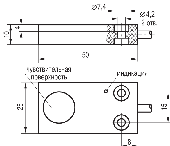
Габаритный чертеж
