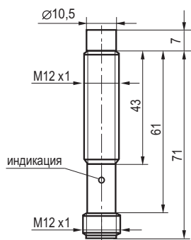
Габаритный чертеж
