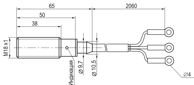
Габаритный чертеж
