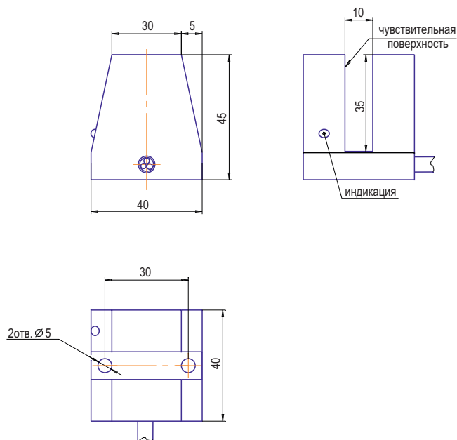
Габаритный чертеж
