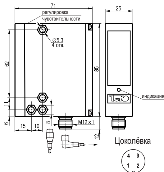
Габаритный чертеж.
