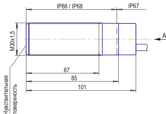
Габаритный чертеж
