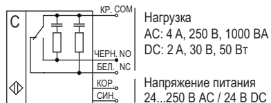
Схема подключения
