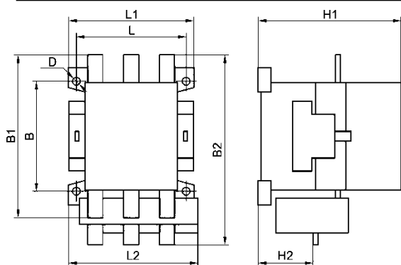
Рисунок 1. Пускатель нереверсивный ПМА-5000, ПМА-6000, IP00
