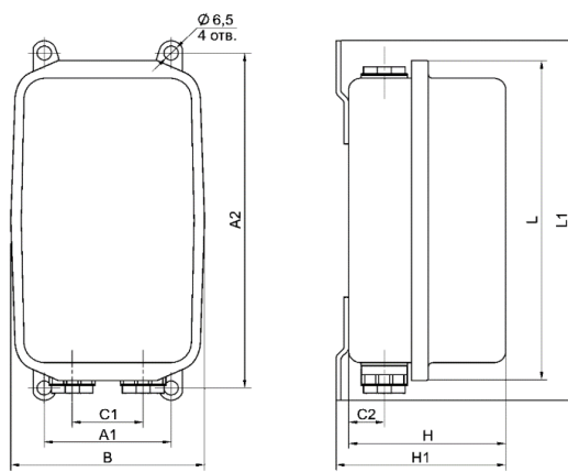
Рисунок 3. Пускатель ПМА-5000, ПМА-6000, IP54
