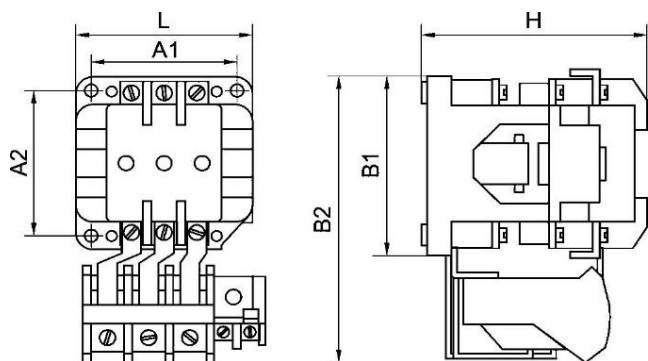
Рисунок 7. Пускатель нереверсивный ПМА-3000. Степень защиты - IP00
