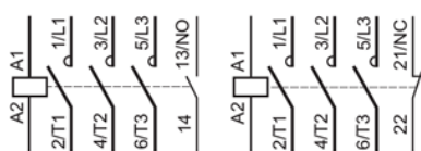
а) контакторы LC1E06...38
