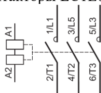
в) контакторы LC1E200...300
