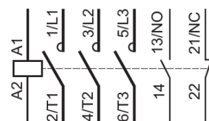
б) контакторы LC1E40...160
