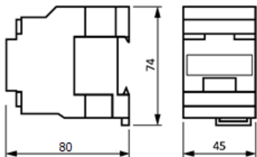
Контакторы LC1E06...18
