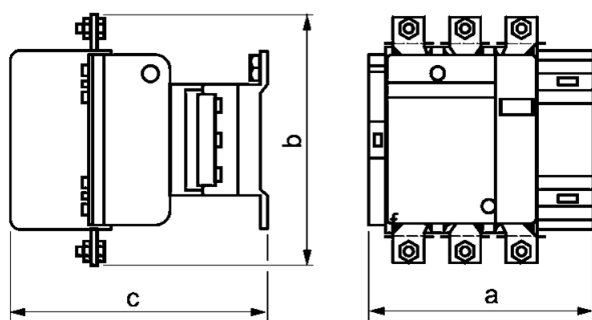
Контактор LC1E200...300
