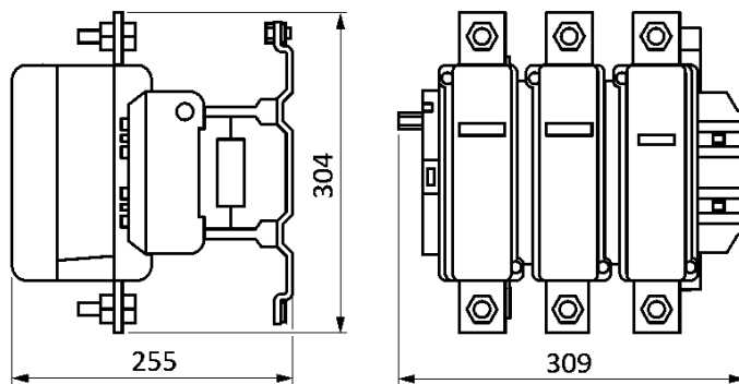
Контакты LC1E630
