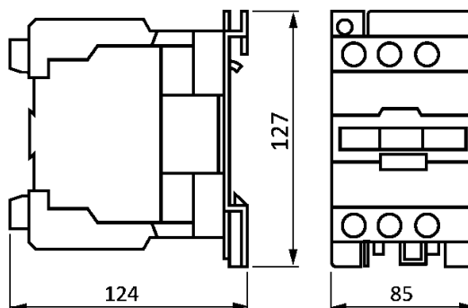
Контакторы LC1E80...95
