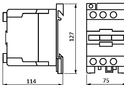
Контакторы LC1E40...65
