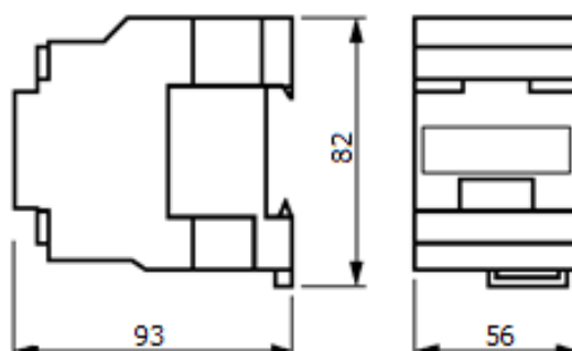
Контакторы LC1E25
