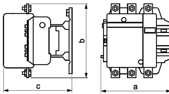
Контакторы LC1E400...500
