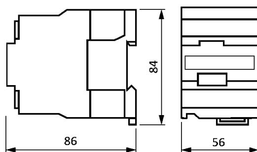
Контакторы LC1E32...38
