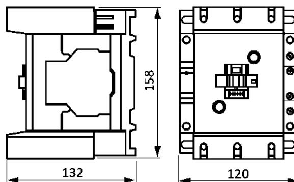
Контакторы LC1E120...160
