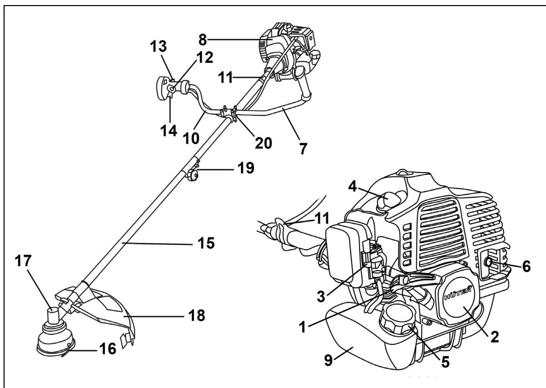
Рис. 1. Общий вид
