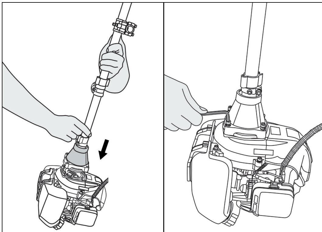
Рис. 6. Установка штанги
