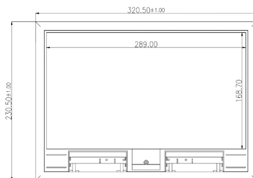
Вид сверху
