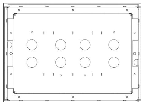
Вид снизу
