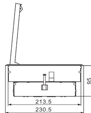
Вид сбоку
