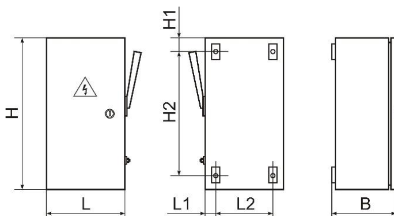
Рисунок 1. Общий вид и габаритные размеры ящиков силовых
