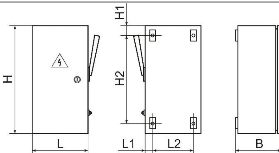
Рисунок 1. Общий вид и габаритные размеры ящиков силовых
