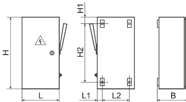
Рисунок 2. Общий вид и габаритные размеры ящиков силовых
