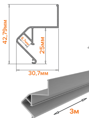
WAP-I-30/43/3000-A
