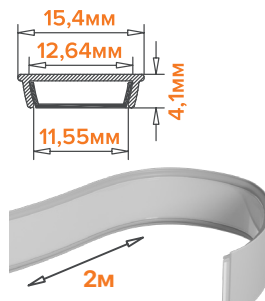
WAP-S-15/4/2000-A
