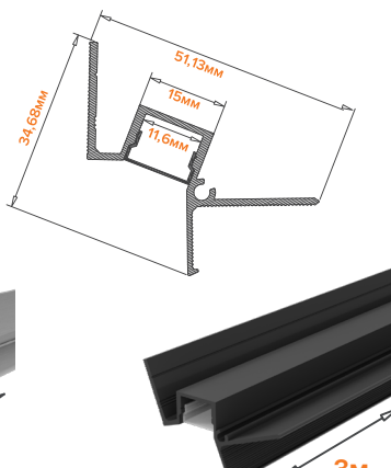
WAP-I-51/35/3000-B
