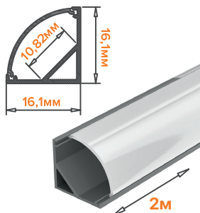
WAP-S-16/16/2000-A
