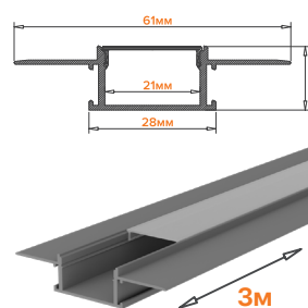
WAP-I-61/14/3000-A
