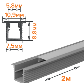
WAP-S-11/9/2000-A
