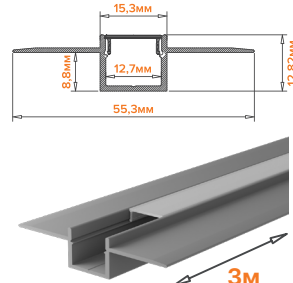
WAP-I-55/13/3000-A
