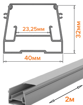
WAP-S-40/32/2000-A
