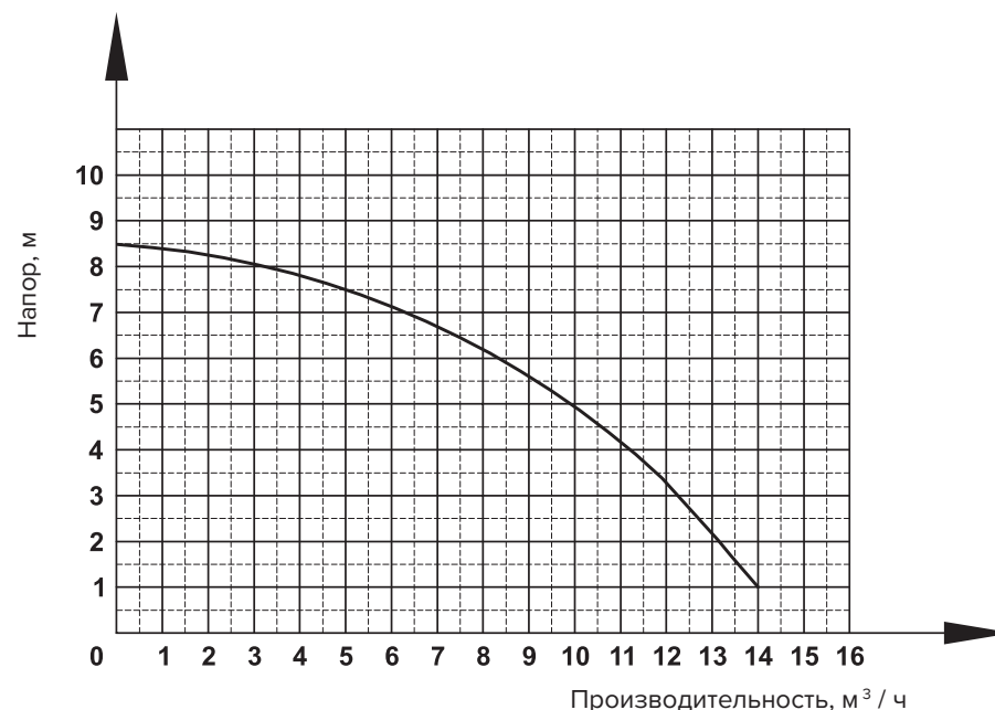
Рисунок 1 — График зависимости производительности насоса от напора
