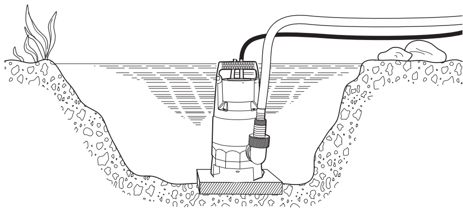
Рисунок 6 — Пример установки насоса на дне водоема
