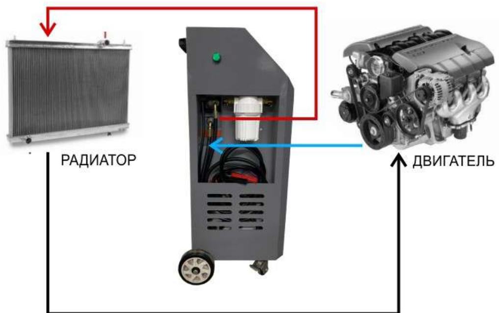
Рис. 3 Схема подключения изделия к системе охлаждения автомобиля
