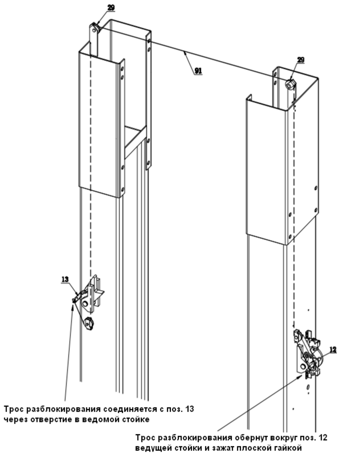
Рис. 15. Система разблокирования кареток
