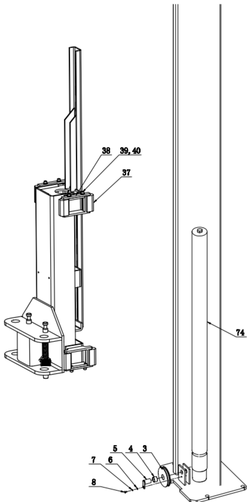
Рис. 11. Узлы и детали подъемника
