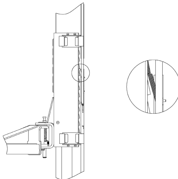
Рис. 1 Замок безопасности
