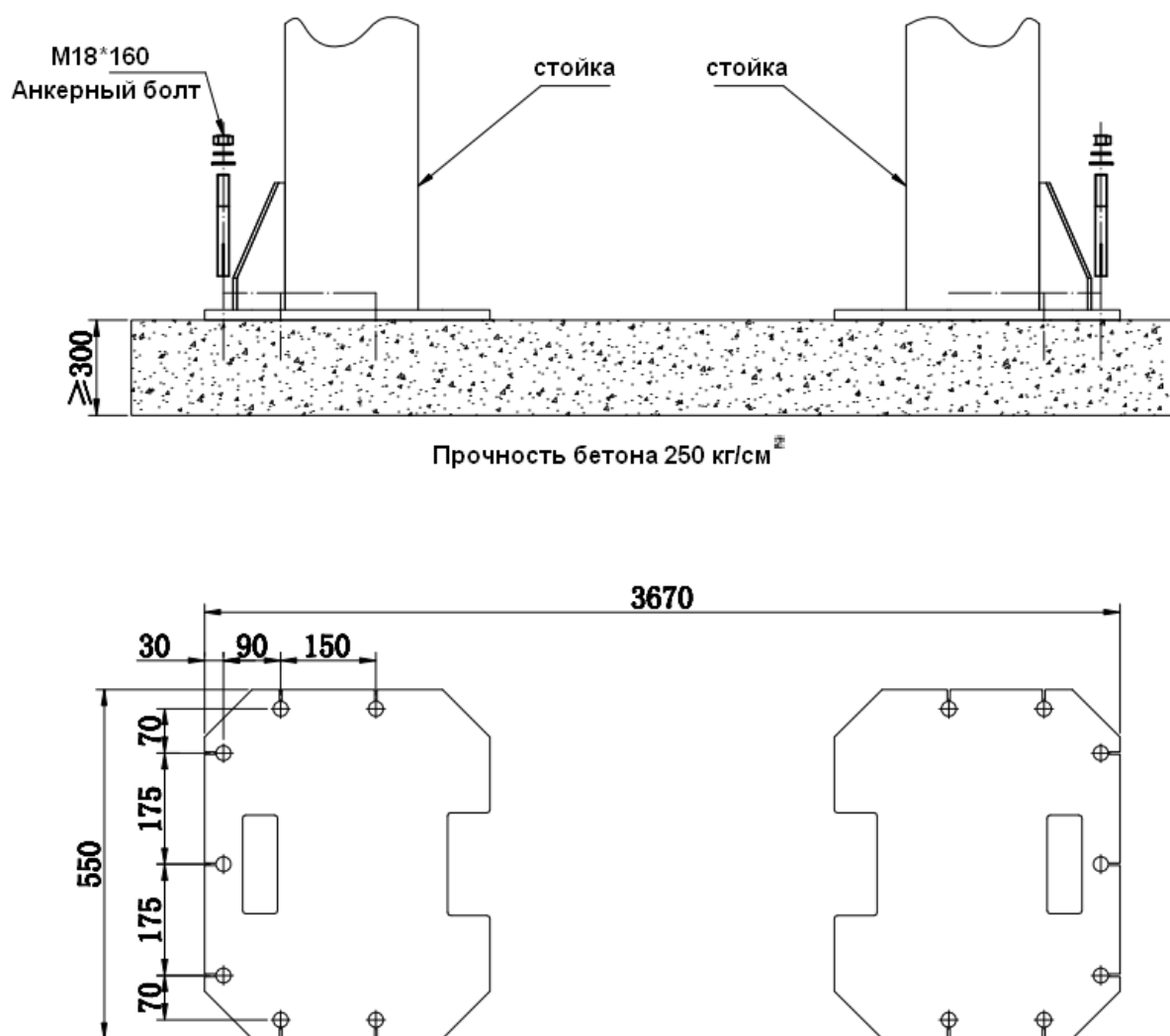
Рис. 2. Фундаментное задание.
