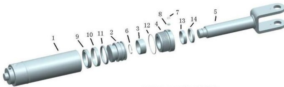
Рис. 6. Гидравлический цилиндр
