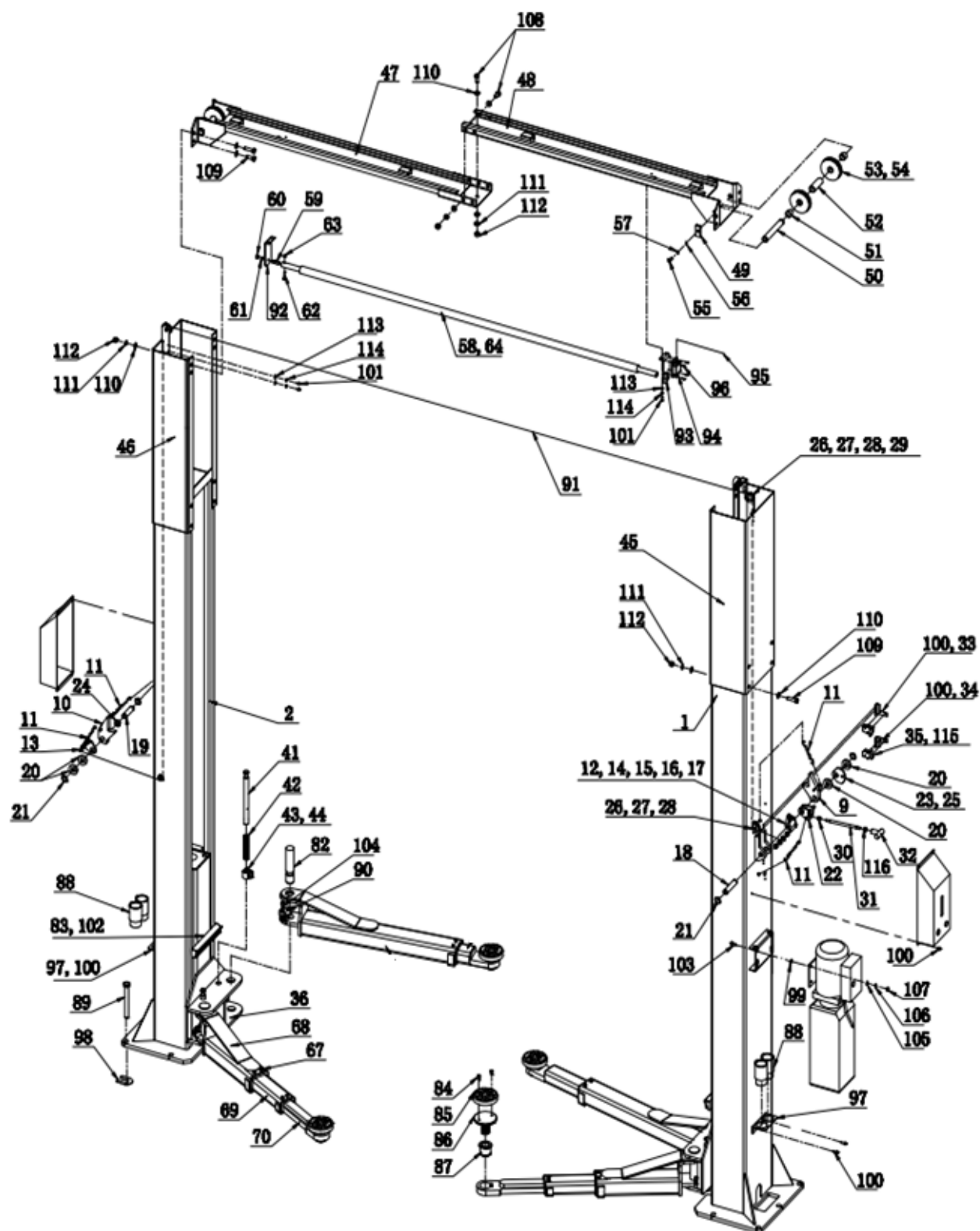
Рис. 10. Узлы и детали подъемника
