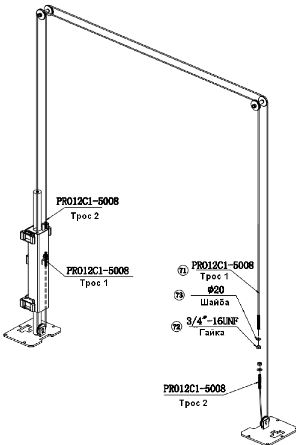
Рис. 14. Система синхронизации кареток
