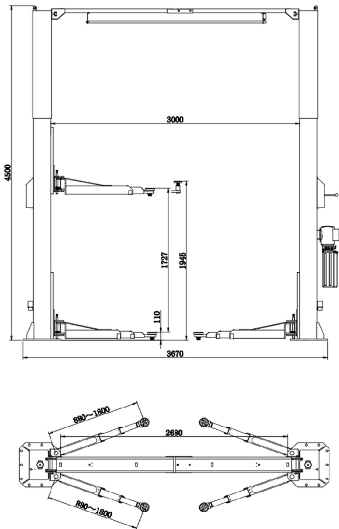
Рис. 3. Габаритные и функциональные размеры.
