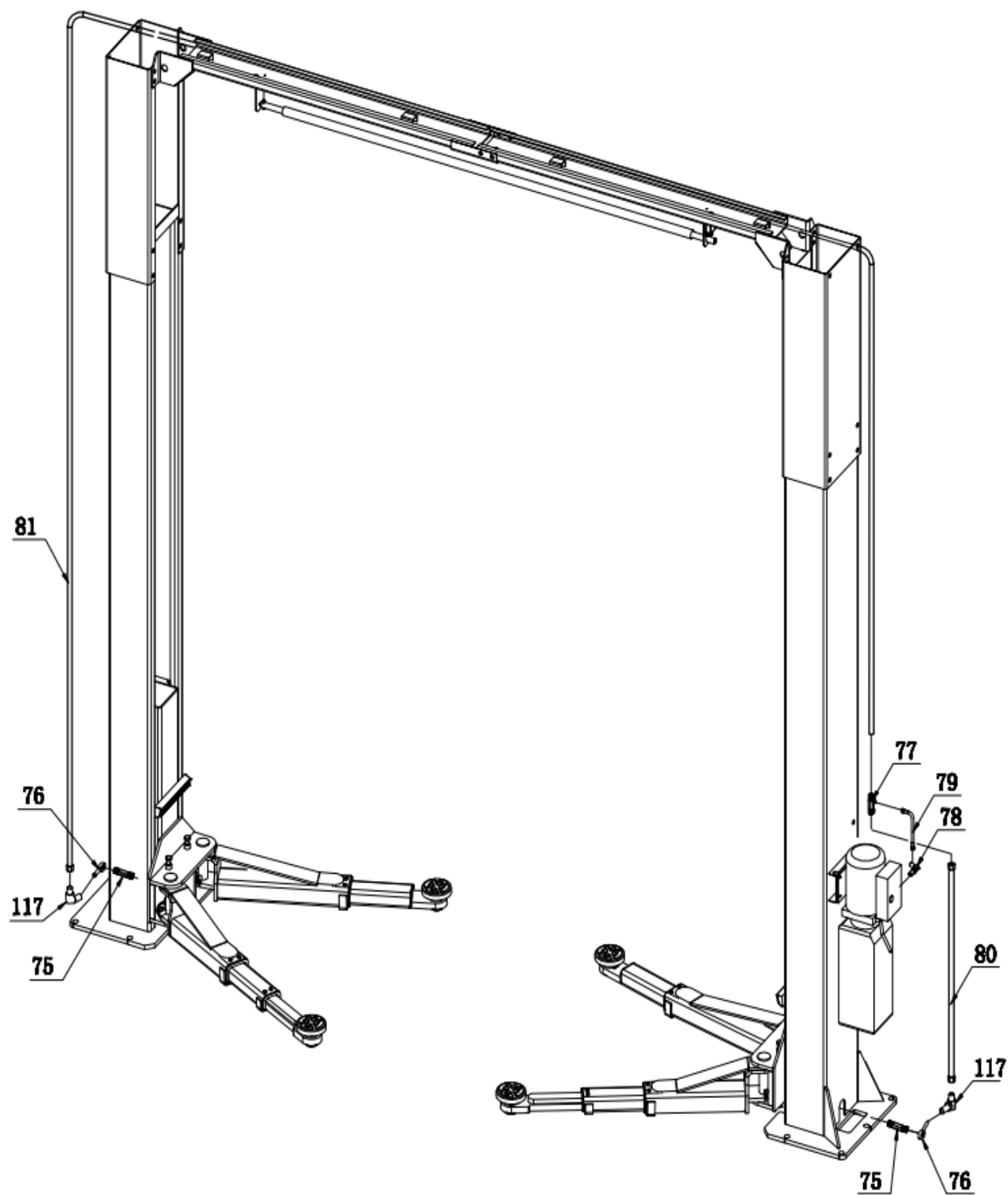
Рис. 12. Узлы и детали подъемника
