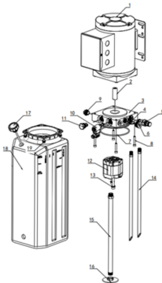
Рис. 7. Насосная станция
