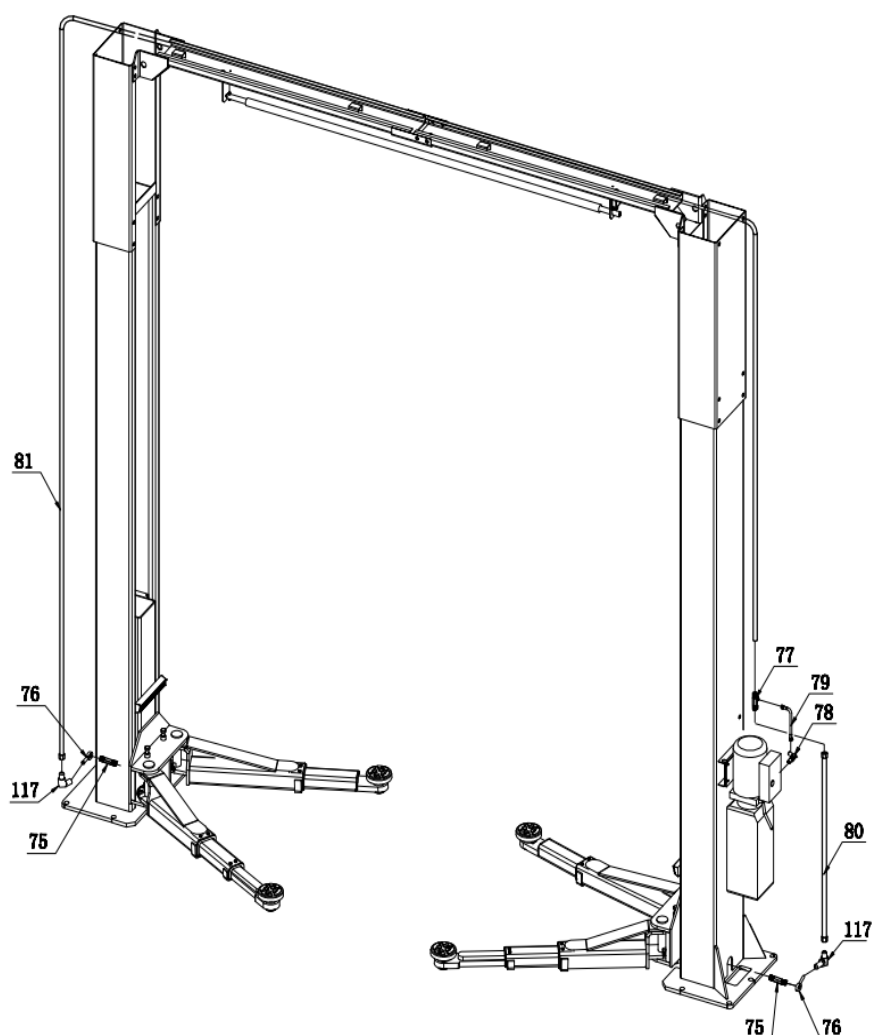
Рис. 8. Монтаж гидравлической системы.
