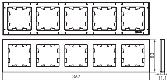
Рис. 8 5-местная рамка, пластик UP1-FP*-05
