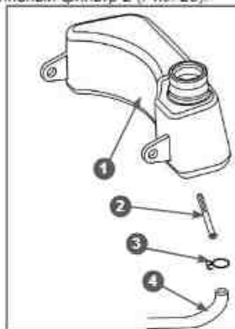
Рис. 23 Обслуживание топливного фильтра
