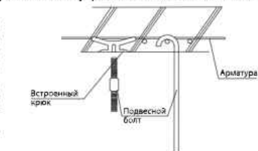
Рисунок 15 - Крепление подвесных болтов к основанию
