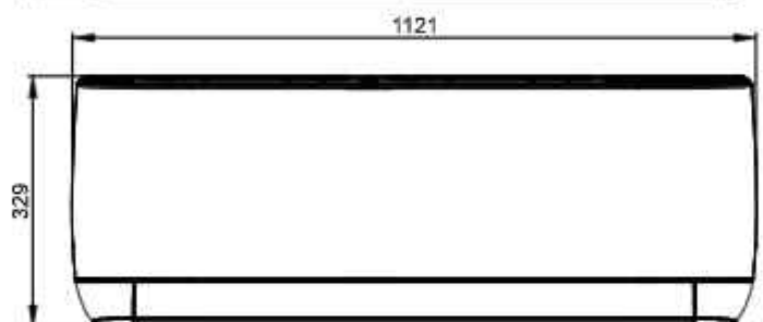
Рисунок 36 - Размеры внутренних блоков настенного типа
