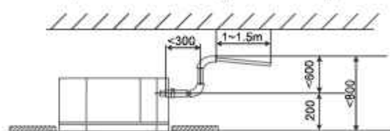
Рисунок 21 - Перегиб дренажной трубки
