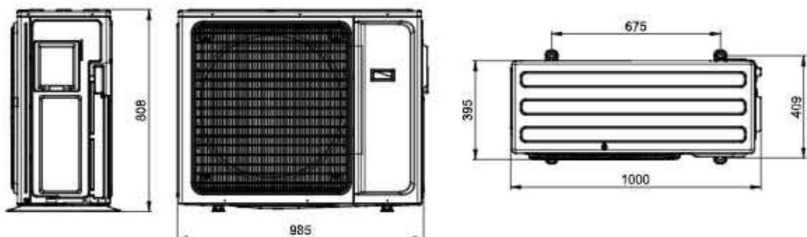
Рисунок 40 - Размеры внешних блоков
