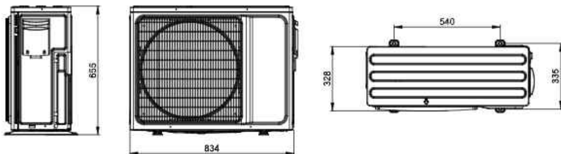
Внешний блок AMSN-21/3AI AMSN-27/3AI
