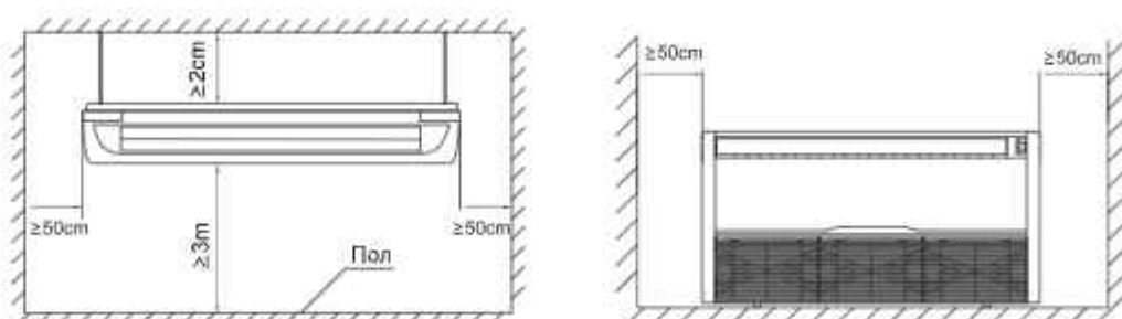
Рисунок 24 - Требования к пространству для установки внутренних блоков напольно-потолочного типа
