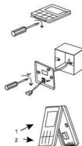
Рисунок 8 - Подключение проводного пульта управления
