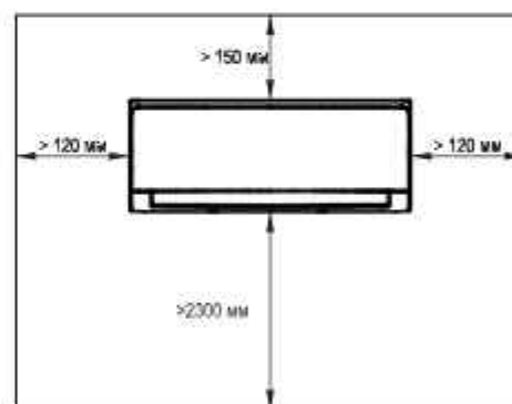
Рисунок 36 - Размеры внутренних блоков настенного типа
