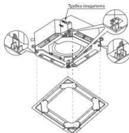
Рисунок 22 - Установка панели
