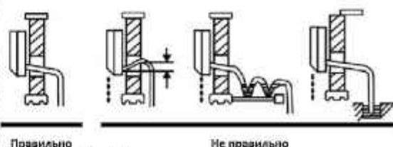
Рисунок 39 - Прокладка дренажа внутреннего блока
