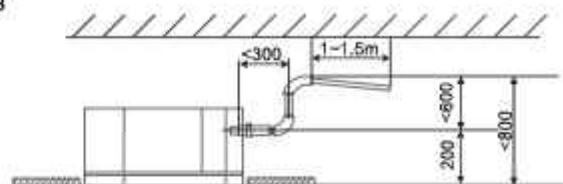
Рисунок 33 - Наклон и перегиб дренажного трубопровода
