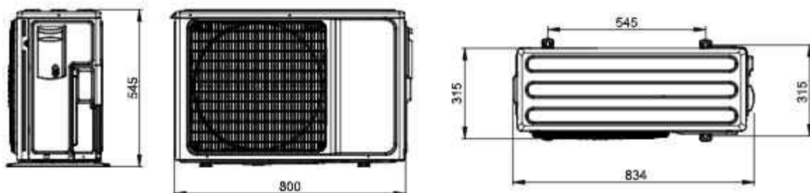
Внешний блок AMSN-14/2AI AMSN-18/2AI
