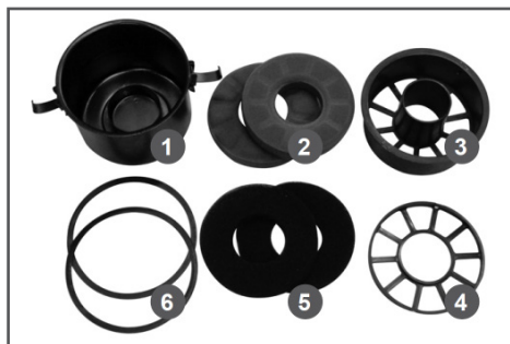
Рис. 17 Воздушный фильтр
