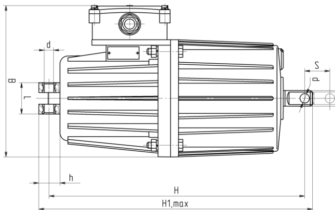
Рисунок 1. Габаритные и установочные размеры ТЭ
