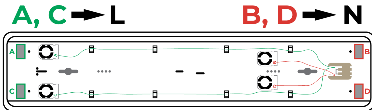
Рисунок 2. Схема подключения светильника
