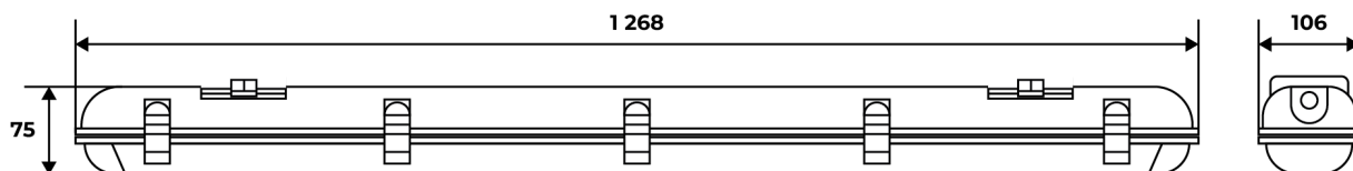
Рисунок 1. Общий вид светильника
