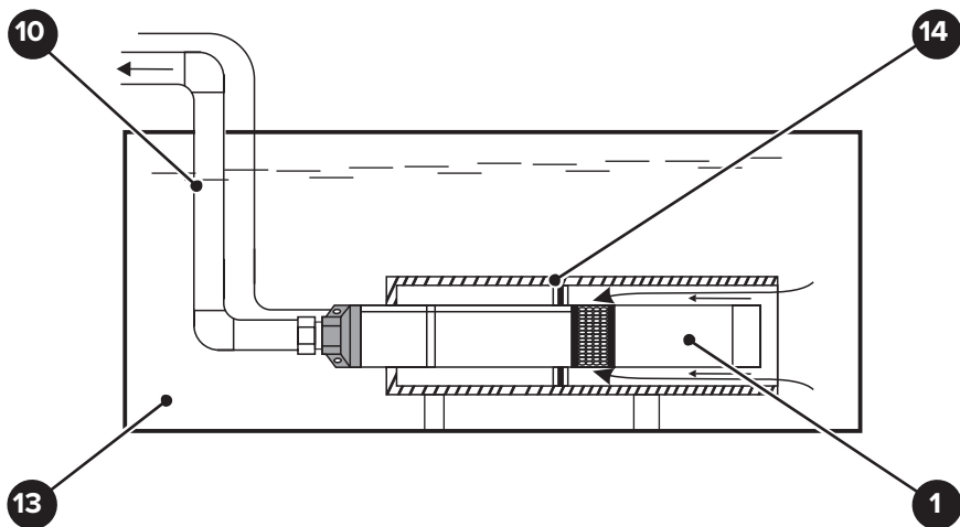
1. Насос 10. Напорный трубопровод 13. Емкость или водоем 14. Дополнительный внешний кожух
