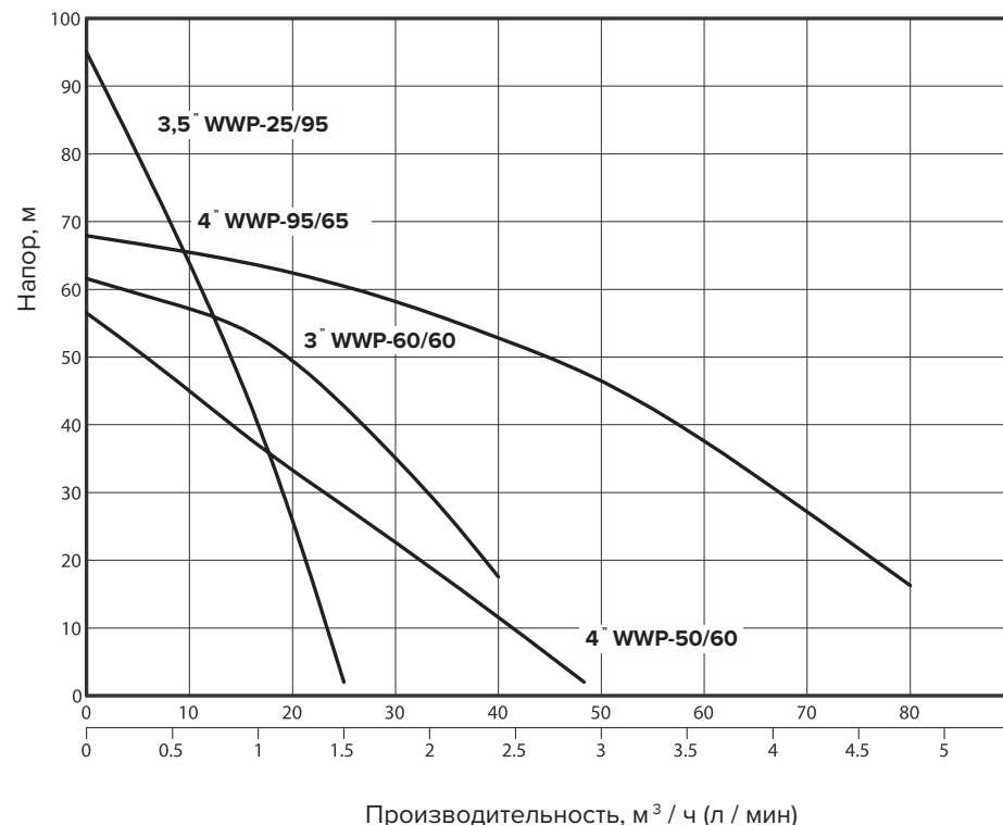
Рисунок 1 — График зависимости производительности насоса от напора
