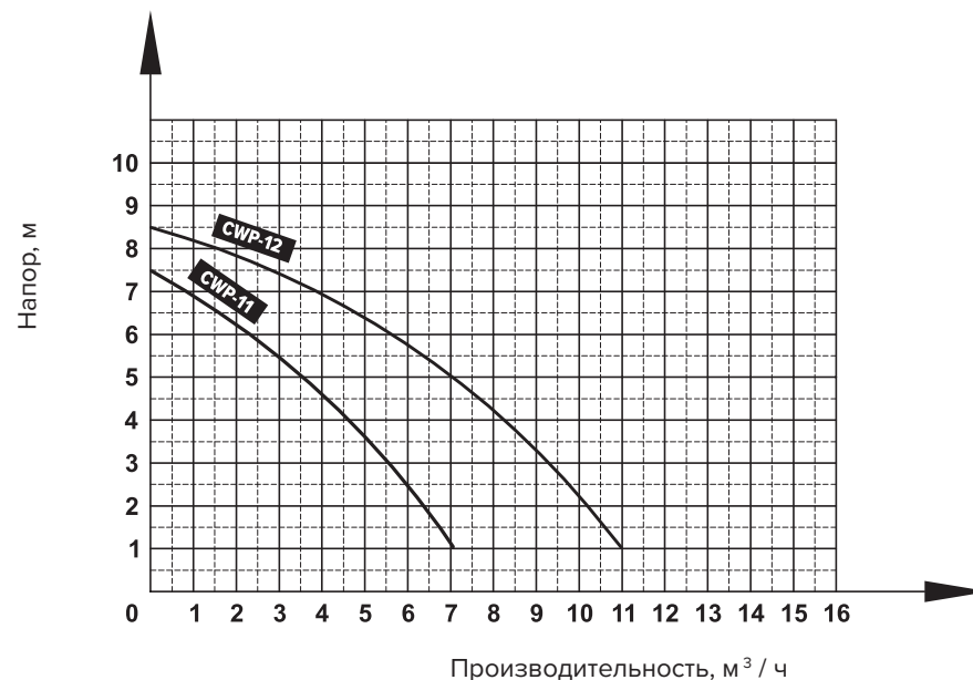
Рисунок 1 — График зависимости производительности насоса от напора
