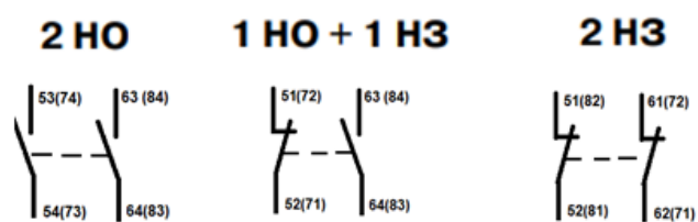
Рис. 5 Принципиальные электрические схемы боковых блок-контактов 3RH1921- EA для S0...3
