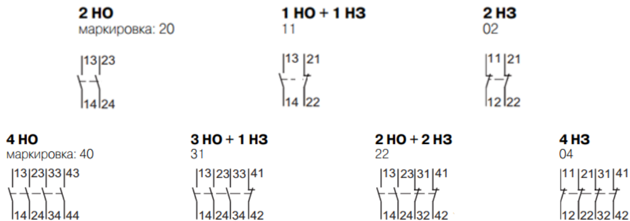
Рис. 4 Принципиальные электрические схемы фронтальных блок-контактов 3RH1921- F для S0...3
