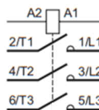
Рис. 2 Контакторы типоразмеров S0... S3
