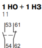
Рис. 2 Контакторы типоразмеров S0... S3
