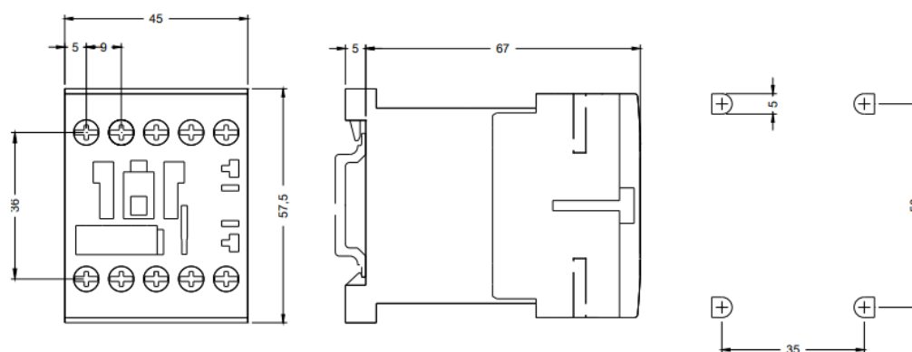
Рис. 6 Габаритные размеры 3RT1015, 3RT1016, 3RT1017 с 3RH1911-1FA
