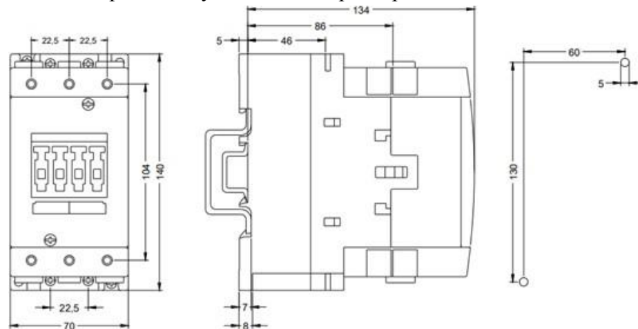
Рисунок 4. Габаритные и установочные размеры 3RT1044, 3RT1045, 3RT1046
