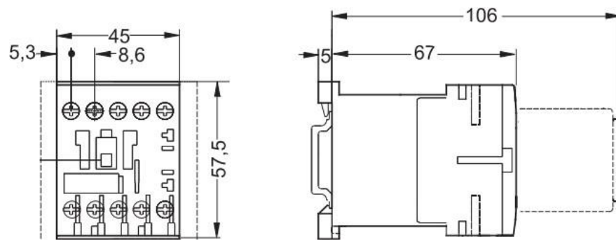
Рисунок 8. Габаритные размеры 3RT1015, 3RT1016, 3RT1017 с 3RH1911-1FA
