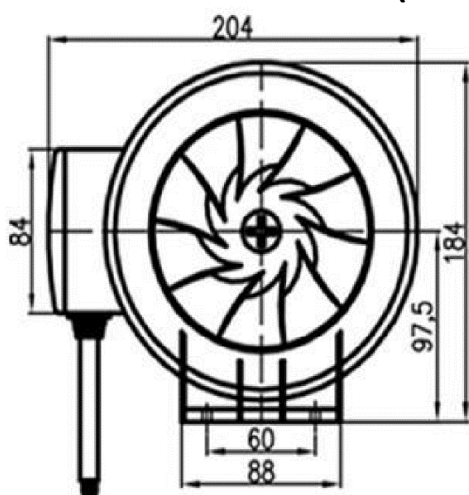
Габаритные размеры Вентилятор канальный осевой VO (AC1) - 125 с пультом (2 скорости)
