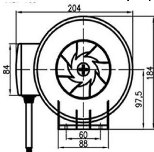
Габаритные размеры Вентилятор канальный осевой VO (AC1) - 100 с пультом (2 скорости)
