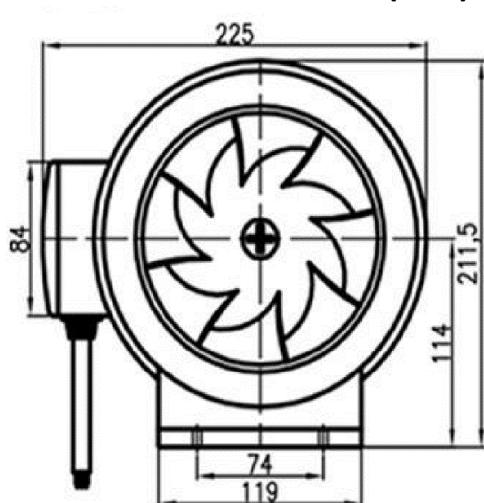
Габаритные размеры Вентилятор канальный осевой VO (AC1) - 160 с пультом (2 скорости)
