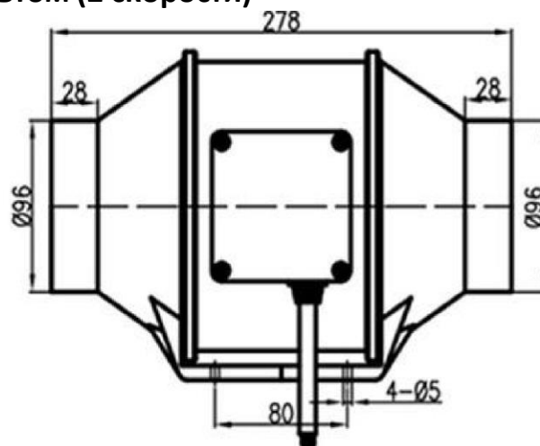
Габаритные размеры Вентилятор канальный осевой VO (AC1) - 100 с пультом (2 скорости)
