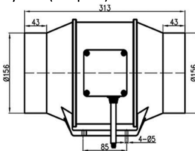
Габаритные размеры Вентилятор канальный осевой VO (AC1) - 160 с пультом (2 скорости)
