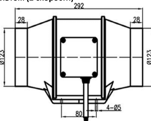
Габаритные размеры Вентилятор канальный осевой VO (AC1) - 125 с пультом (2 скорости)
