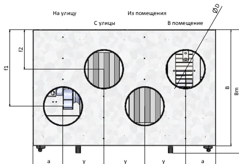
Вид сверху
