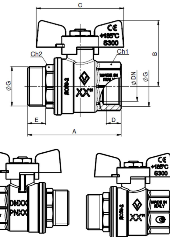
Рис. 2 Габаритные размеры изделия
