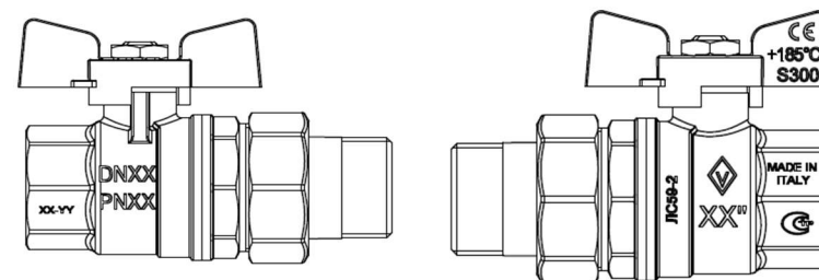
Рис. 2 Габаритные размеры изделия
