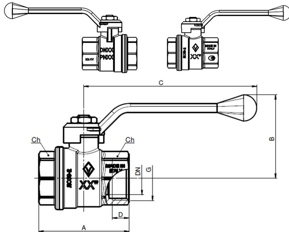
Рис. 2 Габаритные размеры изделия
