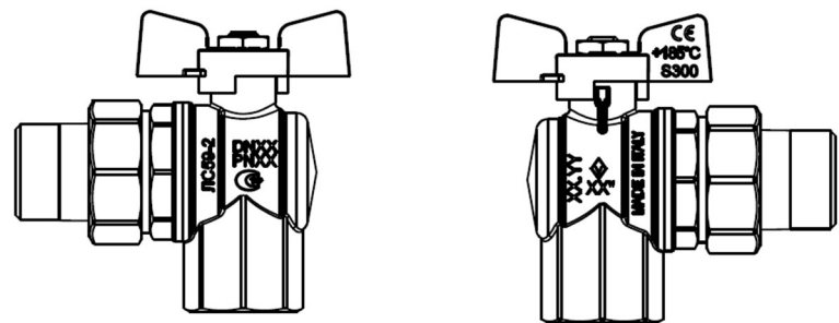
Рис. 2 Габаритные размеры изделия
