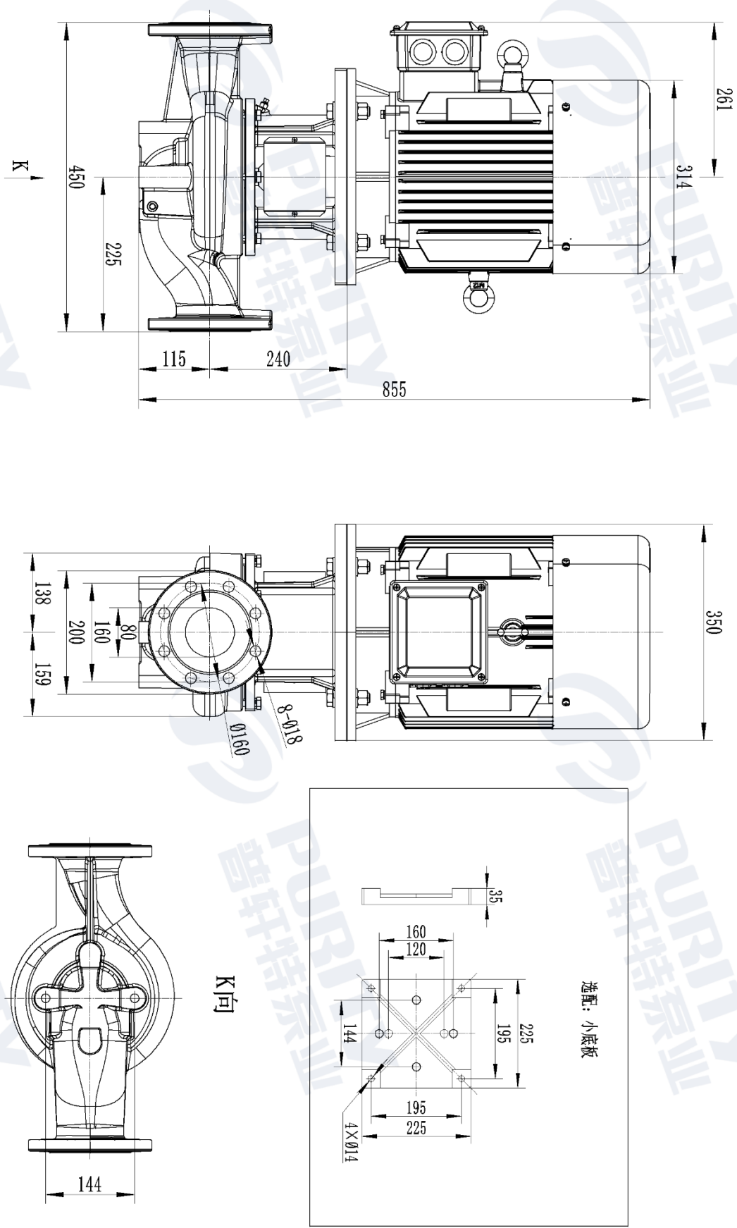
Габаритные и установочные размеры PTD80-32G/2
