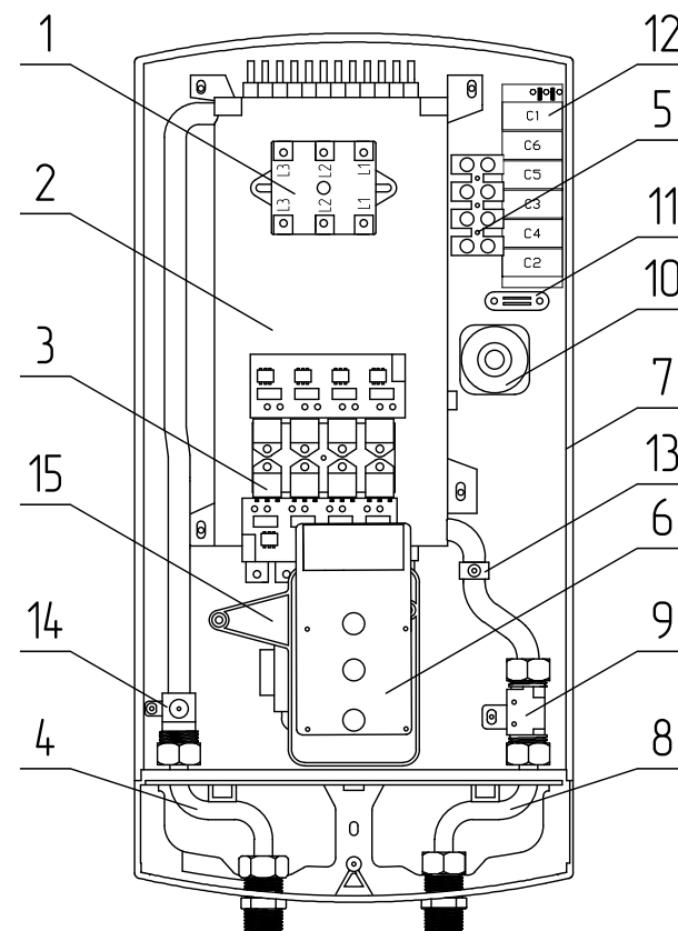
Рис.1 Устройство водонагревателя 9-24 кВт
