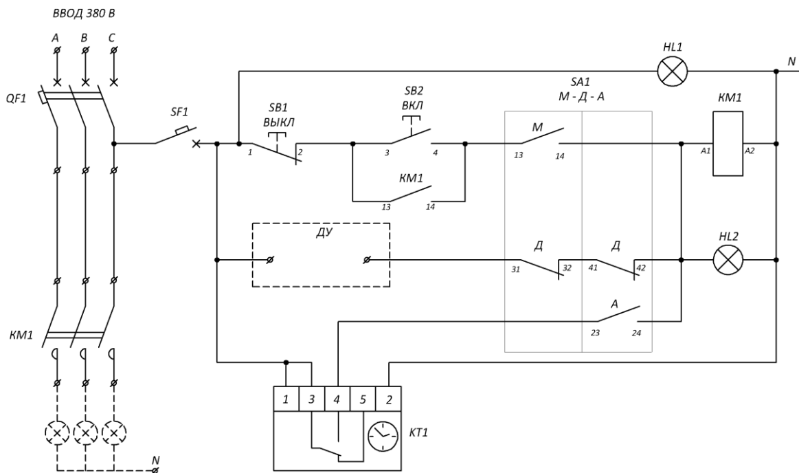
Рисунок 3. Принципиальная электрическая схема ЯУО-9603 (с программатором)
