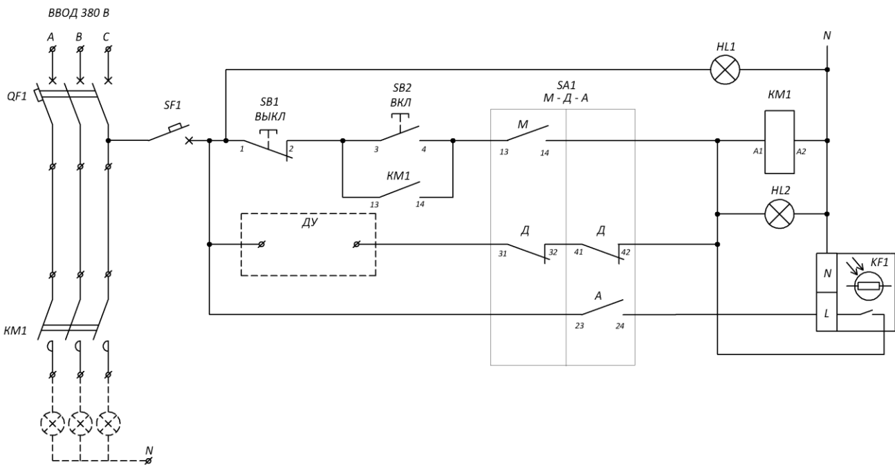
Рисунок 2. Принципиальная электрическая схема ЯУО-9602 (с фотореле)
