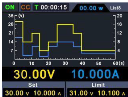
Рисунок 10 - Вывод сигнала по заданным точкам
