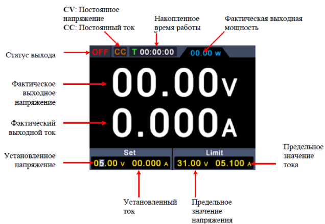
Рисунок 4 - Пользовательский интерфейс
